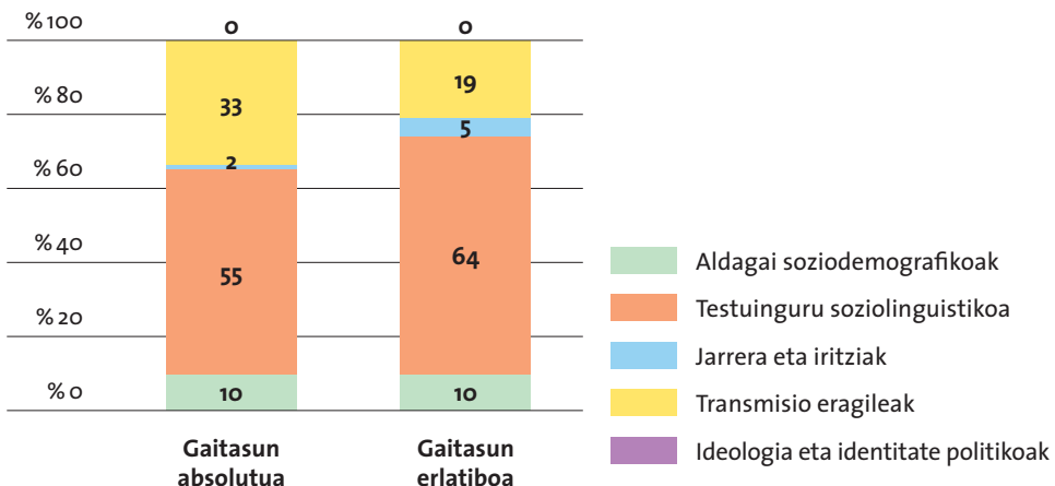
2. grafikoa. Gaitasun linguistiko absolutu eta erlatiboen gaineko aldagai independenteen azalpen gaitasun alderatua (%)
